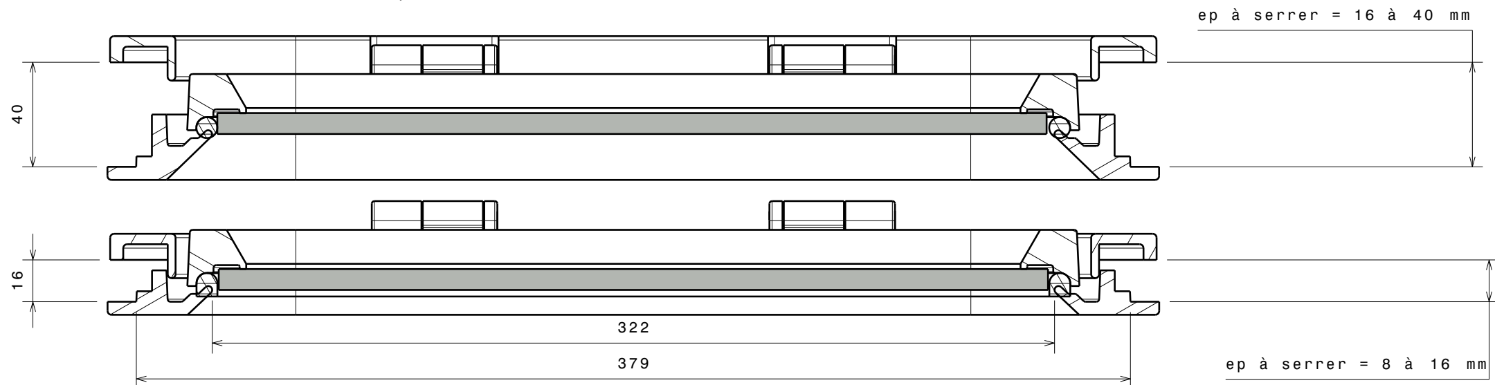
Coupe A-A[2] Ref 99521
