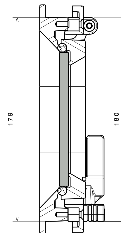
Coupe B-B
