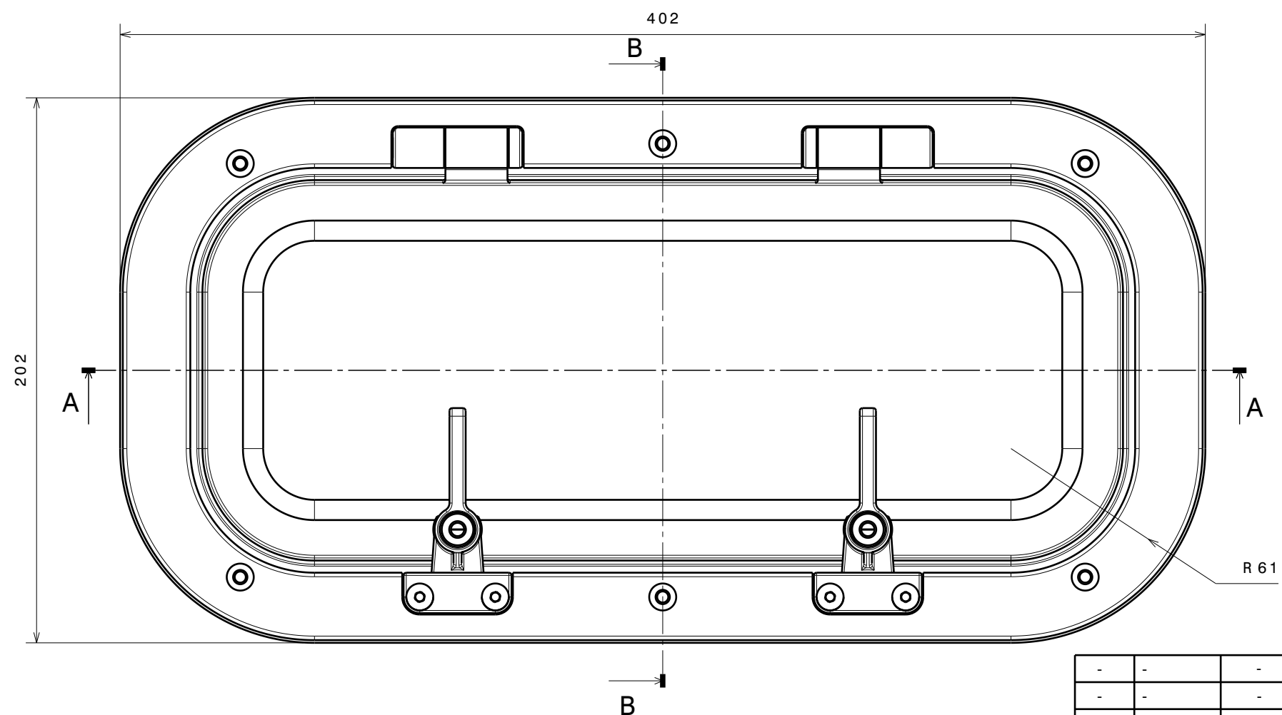
Coupe A-A Ref 115457
