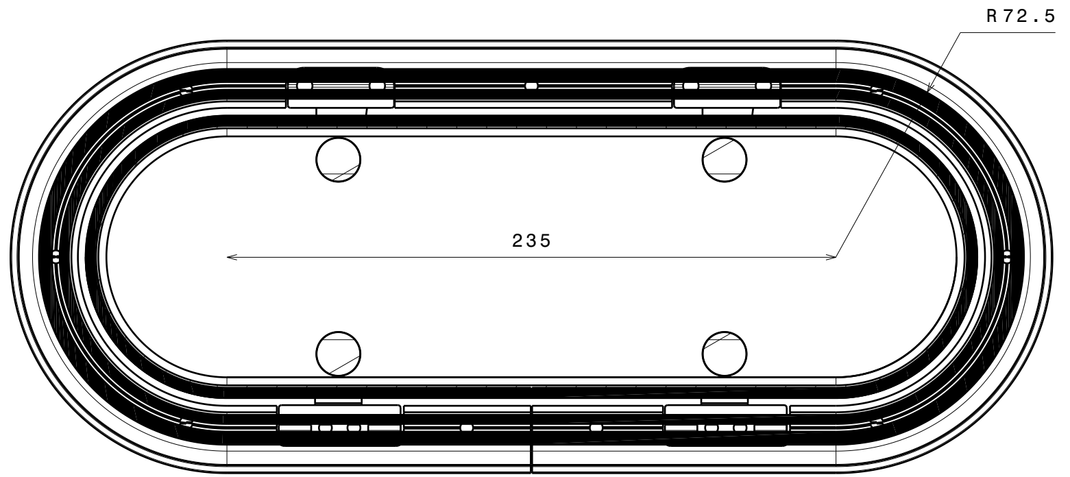
Coupe C-C Echelle : 1:2
