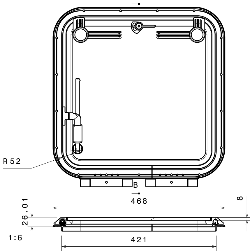
Coupe A-A Echelle : 1:6
