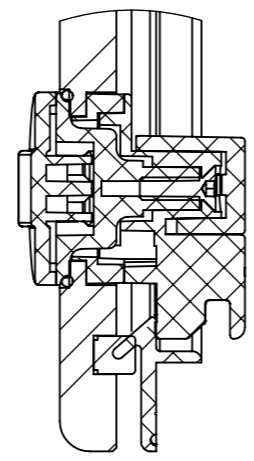
DÉTAIL C ECHELLE 1 : 2
