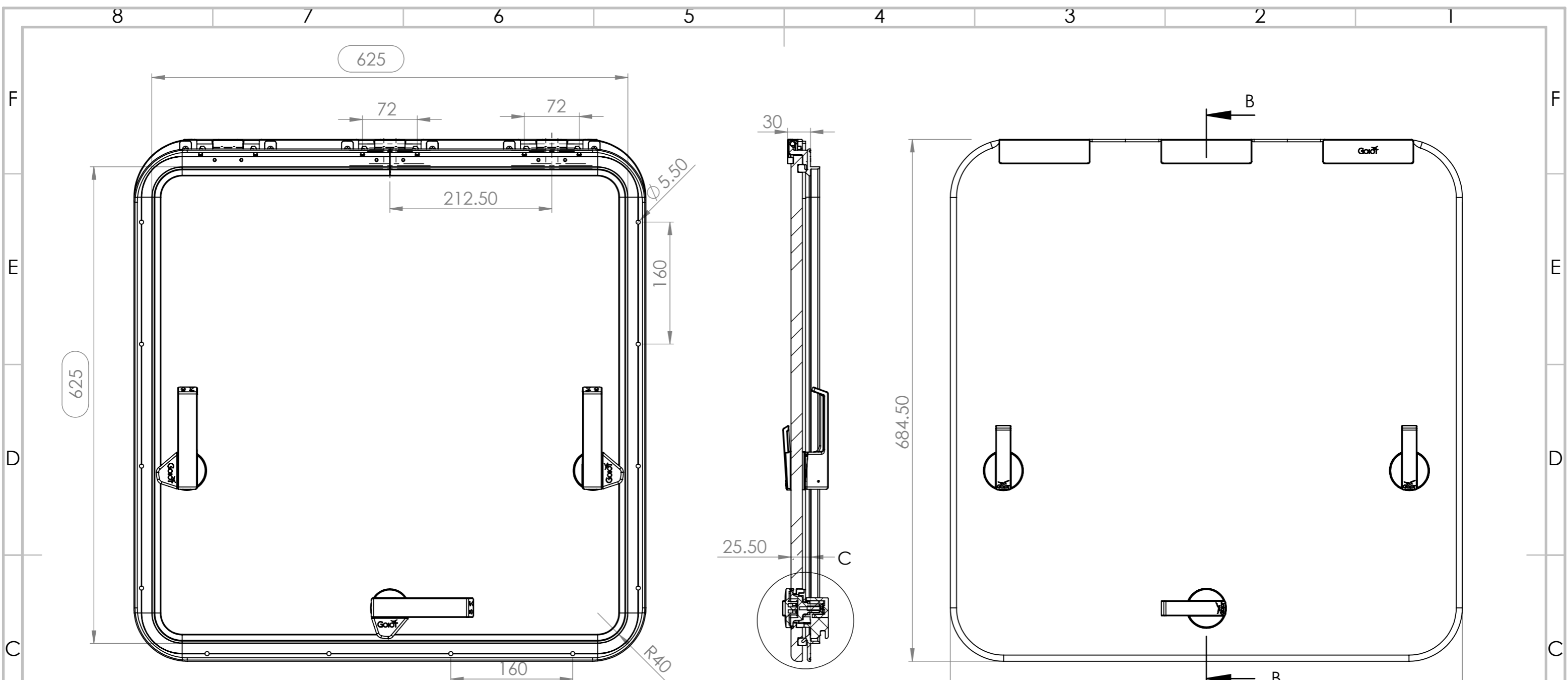
COUPE B-B
